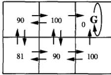
V^*(s) values
